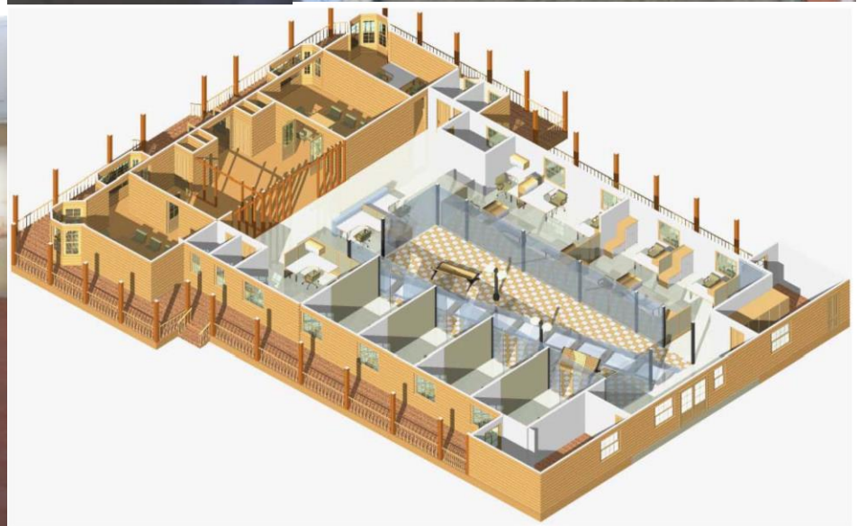
Reconstrucción Casa Huéspedes
